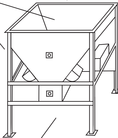
正面
